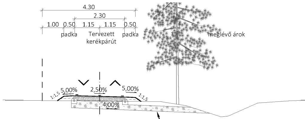
24. ábra 8901 j. út északi oldalán vezetett meglévő fasorral rendelkező szakasz mintakeresztmetszele (M=1:100)
