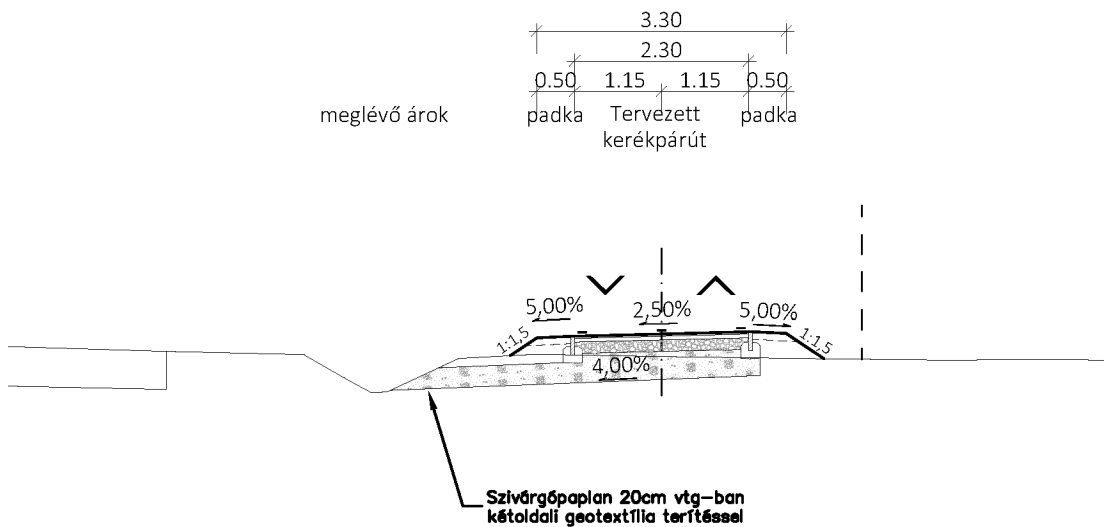
25. ábra 8901 j. út déli oldalán vezetett szakasz mintakeresztmetszele (M=1:100)
