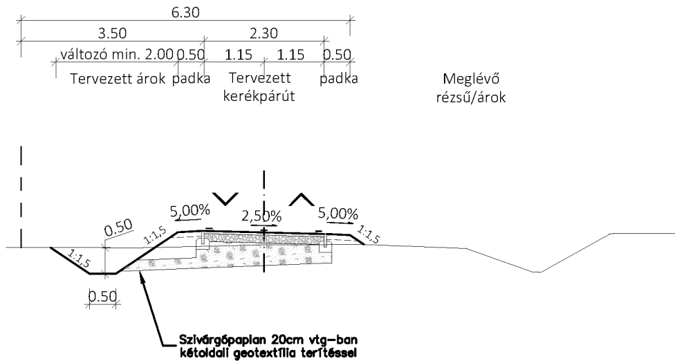
23. ábra 8901 j. út északi oldalán vezetett fasor nélküli szakasz mintakeresztmetszele (M=1:100)
